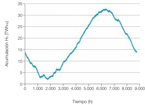
Figura 722. Evolución del estado de carga de la acumulación de hidrógeno con el mix-3b3 dimensionado para cubrir la demanda total del contexto E3.0. SM = 2,25; SF eléctrica = 100%; SF tot = 100%; F dissipada = 0%; C = 3 TWh; CF global = 37,7%; A territorio = 4,3%.
