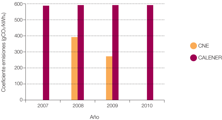
Figura 549. Coeficiente de emisiones del sistema eléctrico nacional, referido a la producción de electricidad, según CNE y CALENER.
