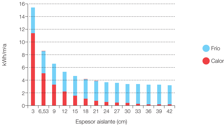
Figura 330. Resultado del estudio paramétrico del efecto del espesor de aislante ( k = 0,04 \text{ W/mK} ) de las paredes sobre la demanda de servicios energéticos de climatización. Cubierta BAU. Suelo BAU para zona D3. Barcelona (C2). El espesor de aislante elegido para el contexto E3.0 es de 18 cm, mientras que el BAU implementa 6,53 cm y el CTE exige 3,54 cm.
