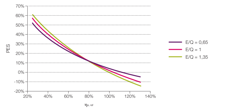
Figura 32. Efecto del \eta_{e,ref} sobre el ahorro de energía primaria para una cogeneración con el 90% de rendimiento total cuando consideramos un proceso de referencia para la generación de calor con una caldera de \eta_{h,ref} = 80\% .
