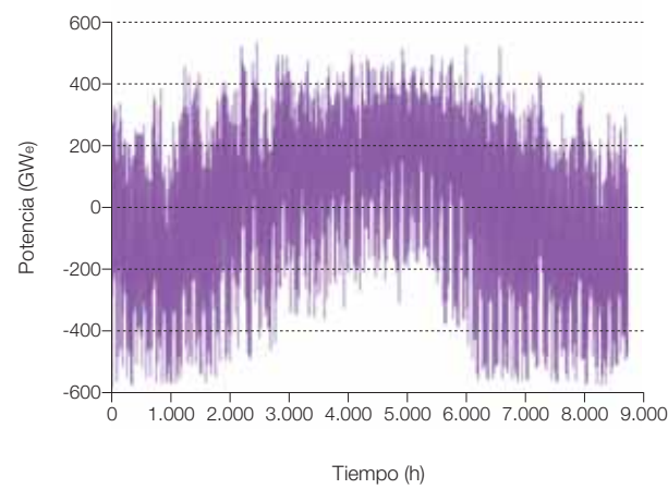
Figura 678. Evolución de las potencias de carga y descarga del sistema de acumulación de hidrógeno para el mix-4b2, dimensionado para la cobertura de la demanda total BAU 2050. SM = 10,6; SF tot = 100% ; F dissipada = 0%; A territorio = 18,9%.
