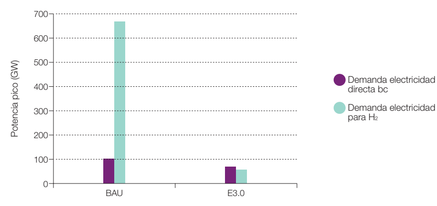
Figura 628. Potencias pico de electricidad directa y electricidad para hidrógeno en los contextos BAU y E3.0 en el año 2050.
