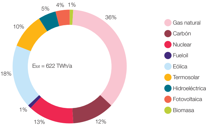
Figura 663. Estructura de la generación eléctrica para el mix BAU en 2050. La generación eléctrica mostrada es en barras de central, e incluyen los efectos del bombeo hidroeléctrico.
