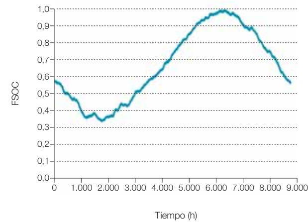
Figura 741. Evolución del estado de carga de la capacidad de acumulación total puesta a disposición del sistema energético para el caso-7, dimensionado para la cobertura de la demanda total en el contexto E3.0 para el año 2050 con participación de la gestión de la demanda e integración de la gestión de acumulación del sistema eléctrico y del sistema de hidrógeno. SM = 2,59 ; SF_{eléctrica} = 100\% ; SF_{tot} = 100\% ; F_{disipada} = 0\% ; CF_{global} = 38,7\% ; C = 82,2 \text{ TWh} ; A_{territorio} = 4,2\% .
