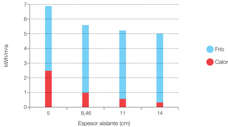
Figura 356. Resultado del estudio paramétrico del efecto del espesor de aislante ( k = 0,04 \text{ W/mK} ) en cubierta sobre la demanda de servicios energéticos de climatización. Pared óptima, suelo BAU. Valencia (B3). Cubierta fría. El valor de aislante elegido para el contexto E3.0 es de 8,46 cm, mientras el contexto BAU implementa 8,46 cm, y el CTE exige 6,16 cm.
