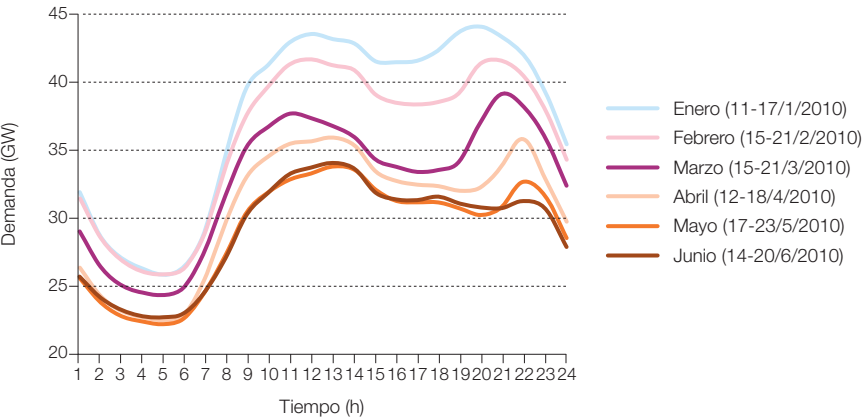
Figura 634. Evolución horaria de la demanda eléctrica durante el martes de una semana tipo para cada uno de los meses del primer semestre del año 2010. Datos ENTSO-E.
