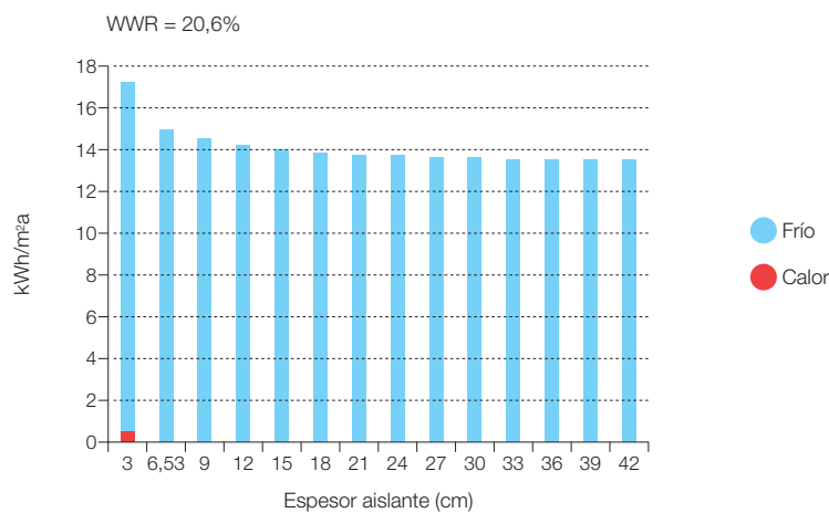
Figura 324. Resultado del estudio paramétrico del efecto del espesor de aislante ( k = 0,04 W/mK) de las paredes sobre la demanda de servicios energéticos de climatización. Cubierta BAU. Suelo BAU para zona D3. Almería (A4). El espesor de aislante elegido para el contexto E3.0 es de 9 cm, mientras que el BAU implementa 6,53 cm y el CTE exige 2,32 cm.
