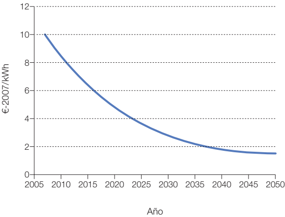
Figura 596. Escenario adoptado para los costes de acumulación de hidrógeno.
