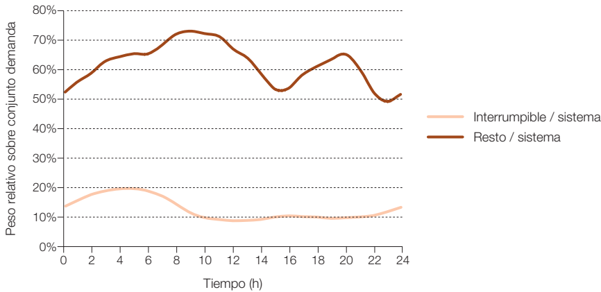
Figura 658. Evolución horaria del peso relativo sobre la demanda eléctrica del sector industrial interruptible y del resto de consumos industriales y de servicios (resto), según resultados del proyecto INDEL.
