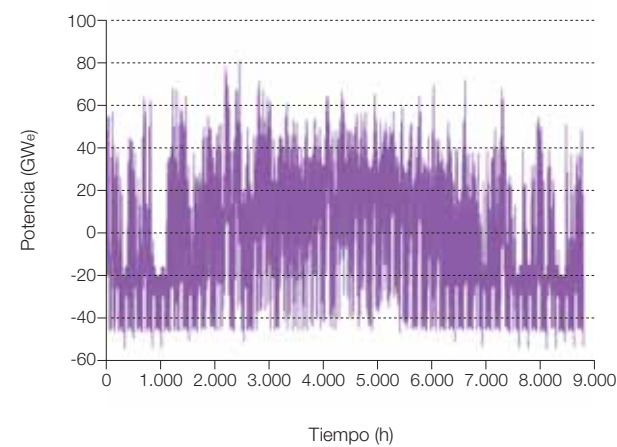
Figura 721. Evolución de las potencias de carga y descarga de la acumulación de hidrógeno con el mix-3b3 dimensionado para cubrir la demanda total del contexto E3.0. SM = 2,25; SF eléctrica = 100%; SF tot = 100%; F dissipada = 0%; C = 3 TWh; CF global = 37,7%; A territorio = 4,3%.
