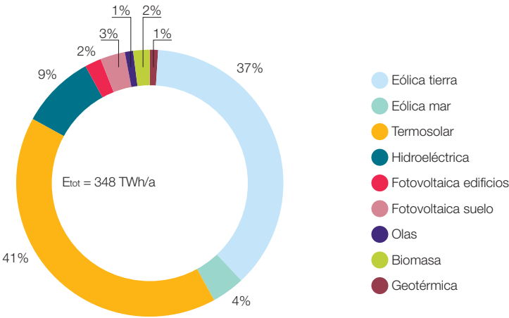
Figura 708. Estructura de la generación en el caso-3b2 dimensionado para cubrir la demanda de electricidad directa (incluye EVs) del contexto E3.0 en el año 2050. SM = 1,55; SF eléctrica = 97,2%; SF tot = 57,6%; F dissipada =15,3%; C = 3 TWh; CF global = 31,5%; A territorio = 3,3%.
