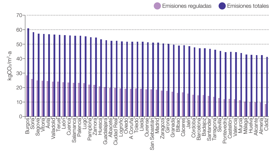
Figura 249. Emisiones de CO 2 medias en viviendas bloque cumpliendo CTE.
