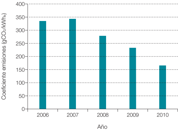
Figura 549. Coeficiente de emisiones del sistema eléctrico nacional, referido a la producción de electricidad, según CNE y CALENER.
