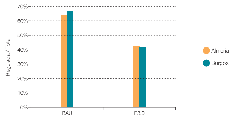
Figura 455. Fracción de consumo de energía regulado respecto al total, para los contextos BAU y E3.0. Hotel.
