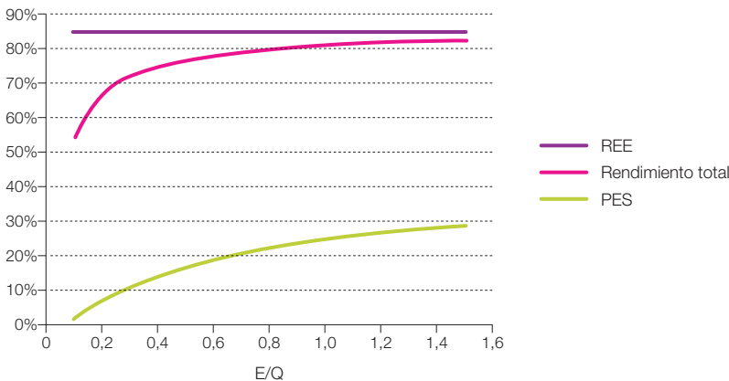
Figura 26. Variación de los distintos indicadores energéticos de una cogeneración con 85% de rendimiento total con la estructura de la demanda (E/Q) cuando se emplean como procesos de comparación \eta_{h,ref} = 90\% y \eta_{e,ref} = 50\% .
