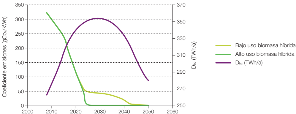
Figura 22. Escenario de evolución del coeficiente de emisiones de CO 2 del sistema eléctrico peninsular asociado a los escenarios de (García-Casals, X, 2009). D bc = demanda en bornas de central.
