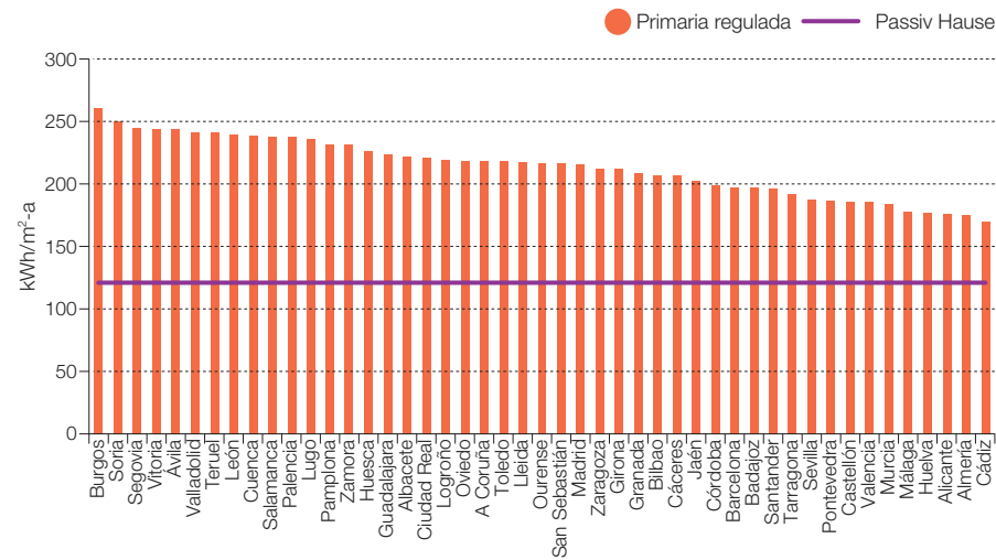
Figura 248. Consumo medio de energía primaria total en viviendas bloque cumpliendo CTE.
