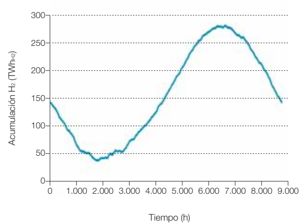
Figura 679. Evolución del estado de carga del sistema de acumulación de hidrógeno para el mix-4b2, dimensionado para la cobertura de la demanda total BAU 2050. SM = 10,6; SF tot = 100% ; F dissipada = 0%; A territorio = 18,9%.
