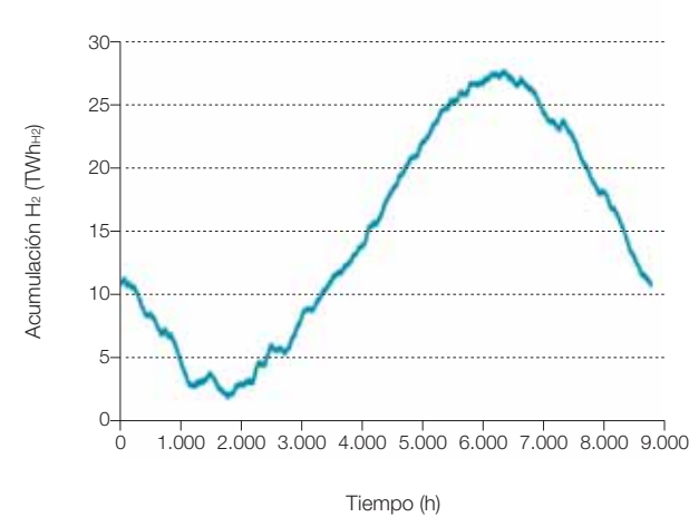
Figura 735. Evolución del estado de carga del sistema de acumulación de hidrógeno para el caso-3b3b, dimensionado para la cobertura de la demanda total en el contexto E3.0 para el año 2050 con participación de la gestión de la demanda. SM = 2,59; SF eléctrica = 100%; SF tot = 100%; F dissipada = 0%; CF global = 38,7%; C = 23,72 TWh; A territorio = 4,2%.
