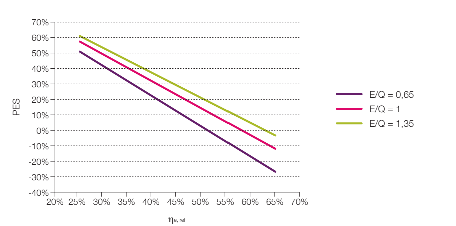
Figura 33. Efecto del \eta_{e,ref} sobre el ahorro de energía primaria para una cogeneración con el 90% de rendimiento total cuando consideramos un proceso de referencia para la generación de calor con una bomba de calor de COP = 3.5.
