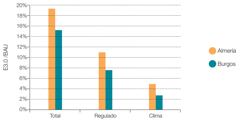
Figura 417. Fracción de consumo de energía total, regulada y de climatización del contexto E3.0 respecto al contexto BAU. Supermercado.
