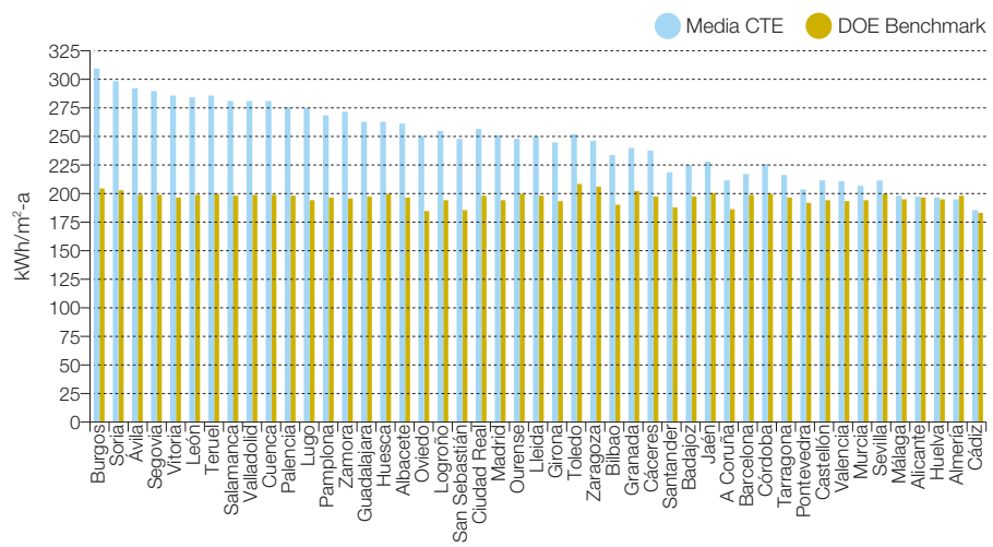
Figura 278. Comparativa de consumo de energía primaria total entre la media de los edificios construidos según CTE (vivienda unifamiliar) y el DOE Benchmark.
