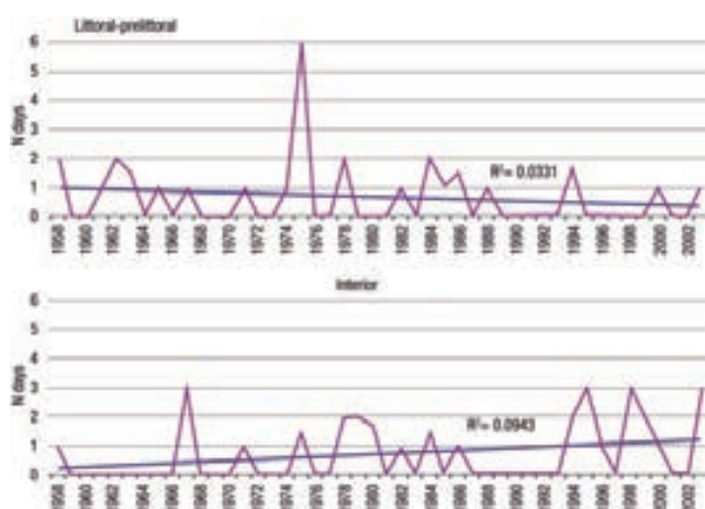
Figura 11. Días con temperatura \geq 40^{\circ}\text{C} . julio. Fuente: Summer temperature trends in a Mediterranean Area (Valencia Region). (Miró et al. 2006) 9 .
