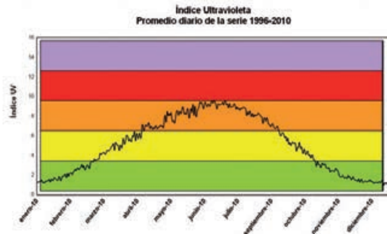
Figura 12.- Índice ultravioleta. Promedio diario de la serie 1996-2010. Fuente: Elaboración propia a partir de los datos de la Agencia Española de Meteorología (AEMET).
