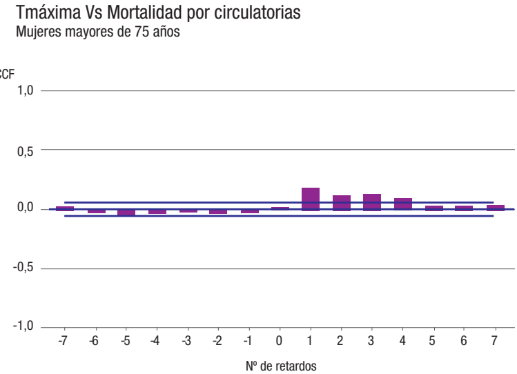
Figura 3. Función de correlación cruzada (FCC) entre la mortalidad por causas circulatorias en mujeres mayores de 75 años en Madrid y la temperatura máxima diaria.
