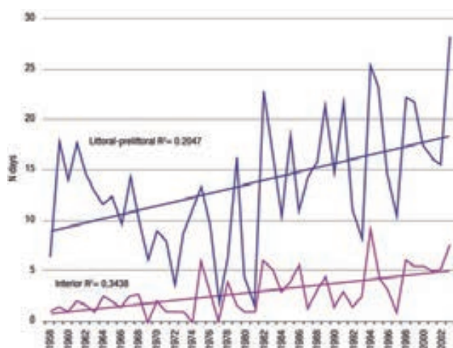
Figura 9.- Número de días de calor persistente en la Comunitat Valenciana. Mes de Julio. Fuente: Summer temperature trends in a Mediterranean Area (Valencia Region). (Miró et al. 2006) 9 .
