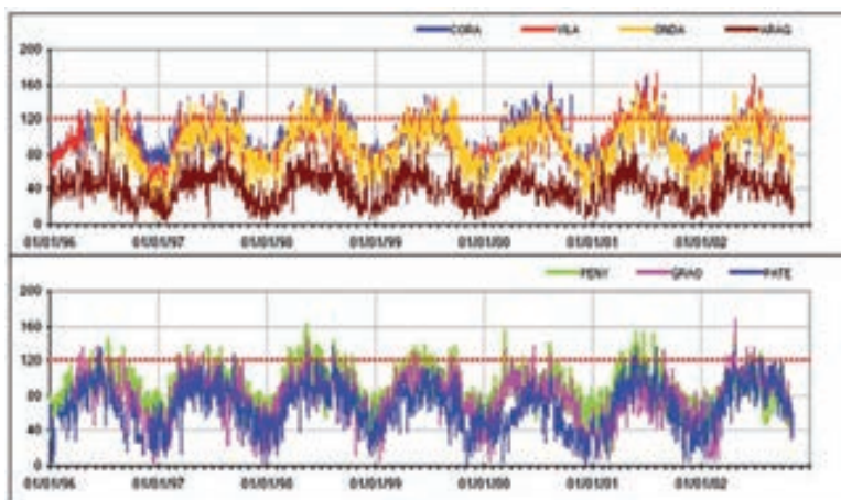
Figura 10.- Máximos de las medias móviles de 24 h en las estaciones señaladas. Se puede observar que los valores de la directiva europea para los daños a la salud (superiores a 120 \mu\text{g}/\text{m}^3 promedio de 24 h, un máximo de 25 días año) solo se cumplen en las estaciones urbanas (ARAGON, PATERNA) dominadas por las emisiones de \text{NO}_x de los vehículos. A sotavento de las ciudades durante el día (ver Figura 6) la directiva no se cumple, ni se puede cumplir en verano en ningunas estaciones con emplazamientos similares situadas alrededor de la Cuenca Mediterránea Occidental, dado el carácter recirculatorio de las masas de aire en esta región durante la mayor parte del año (DOUE 2004). En el gráfico superior se puede observar una tendencia a la subida de los promedios de 24 h por encima de los 160 \mu\text{g}/\text{m}^3 .
