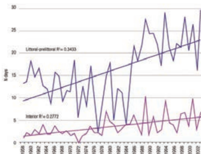
Figura 12. Días con temperatura \geq 40^{\circ}\text{C} . agosto. Fuente: Summer temperature trends in a Mediterranean Area (Valencia Region). (Miró et al. 2006) 9 .
