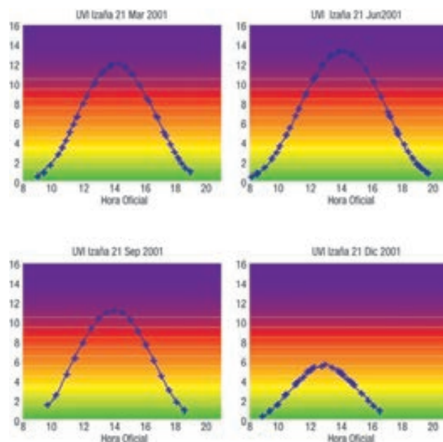
Figura 11.- Variación diaria del IUV observado en Izaña (Tenerife). Fuente: Carreño V, Redondas A, Cuevas E 3 .
