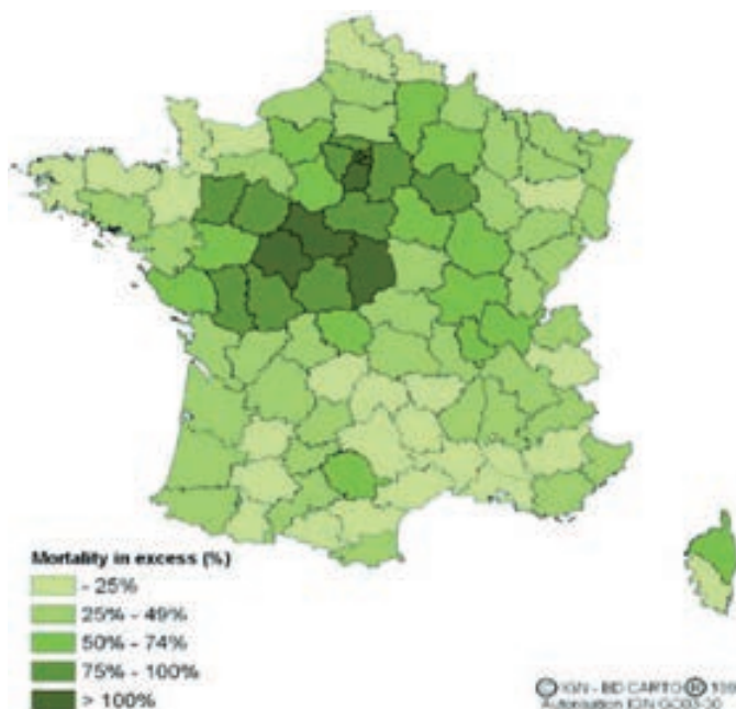
Figura 3.- Los efectos de la ola de calor de 2003 en Francia. Fuente: IPCC, 2007.
