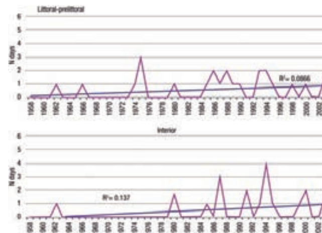
Figura 12. Días con temperatura \geq 40^{\circ}\text{C} . agosto. Fuente: Summer temperature trends in a Mediterranean Area (Valencia Region). (Miró et al. 2006) 9 .
