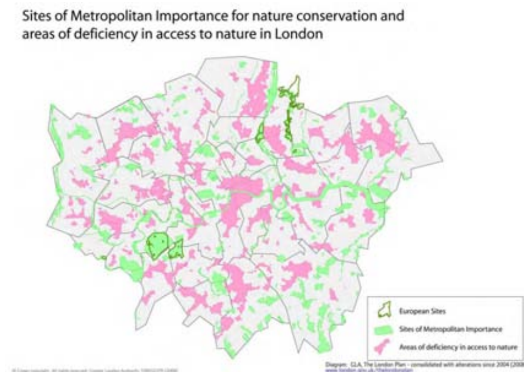
Figura 11.5: Áreas de importancia metropolitana para la preservación de la naturaleza y áreas de deficiencia en el acceso a la naturaleza en el Gran Londres
