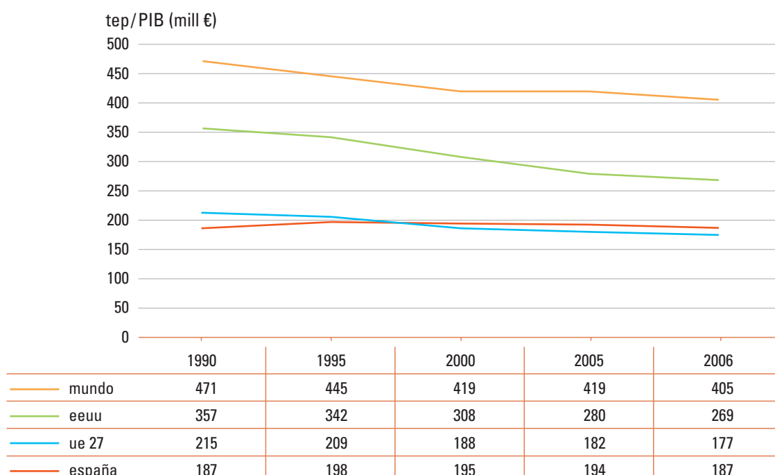
Figura 4: Intensidad energética (toneladas equivalentes de petróleo por millón de euros de producción).
